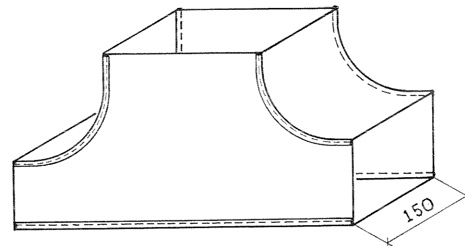
T-förgrening
